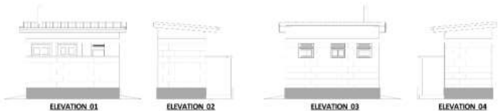
ELEVATION 01
