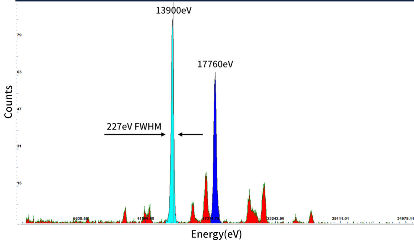
图3: 镅241 (227eV)
