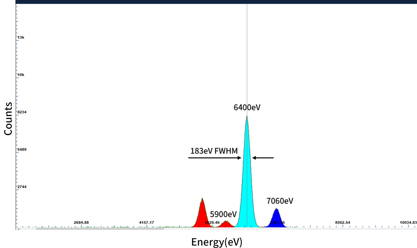
图1：铁（183eV）
