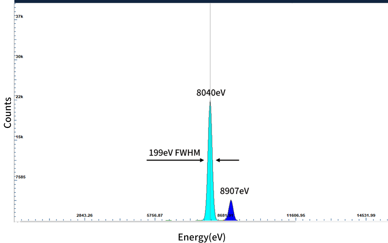
图2：铜（199eV）
